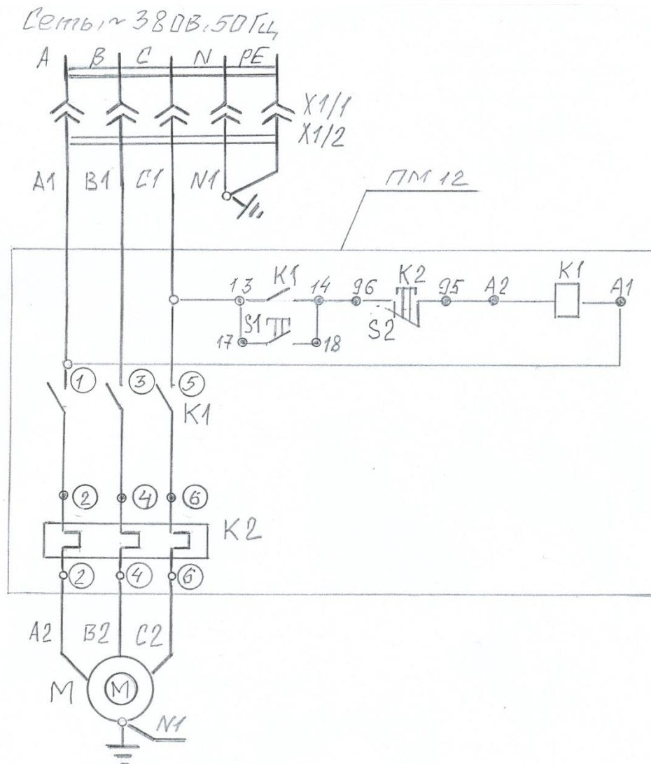
Рисунок 1 – Схема электрическая принципиальная машины СО-300
