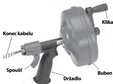
Obrázek 1 – Čistič odpadů Power-Spin
