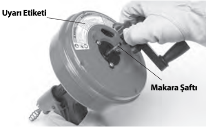
Şekil 2 - Power-Spin'den Krank Tutacağına Çıkarılması
