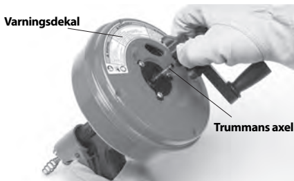
Figur 2 – Borttagning av veven från Power-Spin
