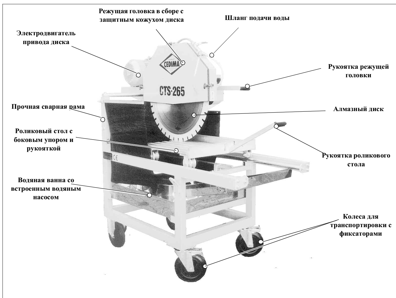
Рис 2.1 Настольная пила CTS•265
