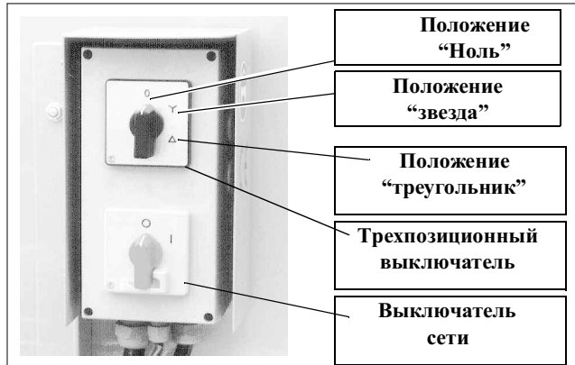
Рис 3.13 Выключатели настольной пилы
