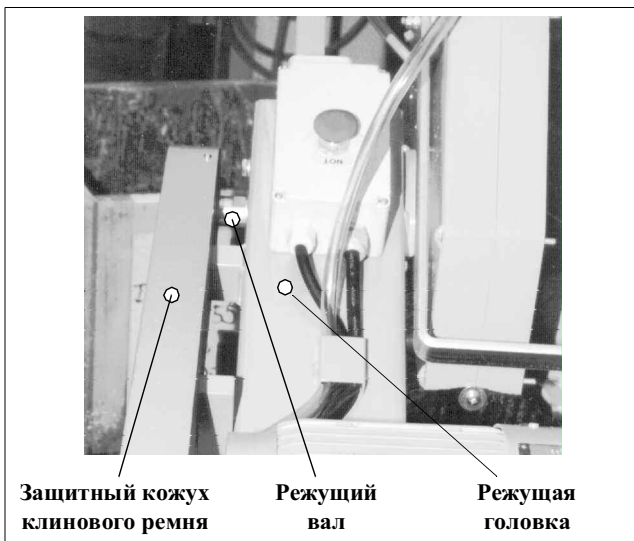
Рис 3.8 Место фиксации режущего вала
