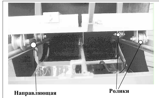
Рис 3.3 Установка роликового стола
