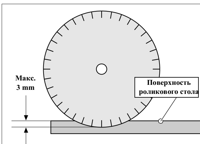
Рис 3.11 Ограничение глубины резания
