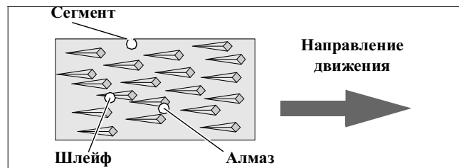
Рис 3.10 Свойство алмазов
