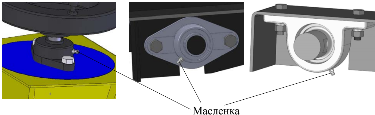
Рисунок 14 – Техническое обслуживание корпусных подшипниковых узлов
