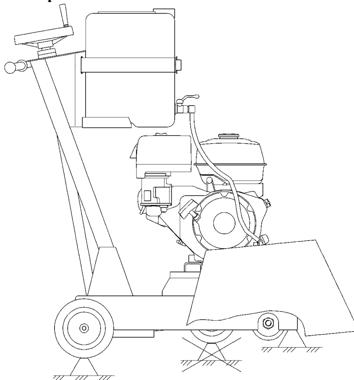
Рисунок 15 – Схема установки разделщика при транспортировании
